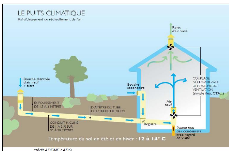
Figure 135 Exemple d'un puits climatique
