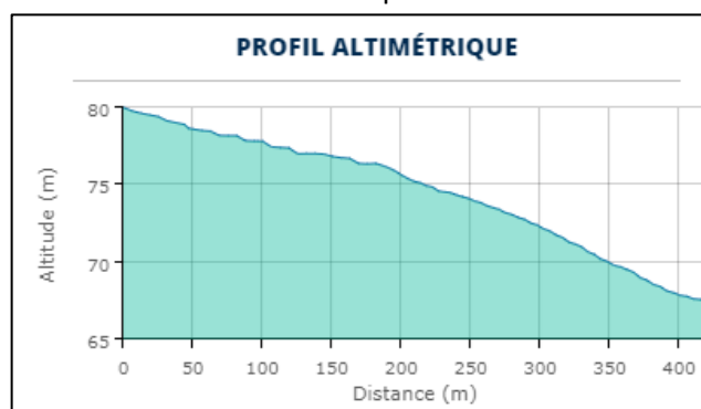
Figure 113 : Profil altimétrique de l'axe de ruissellement N°3.
