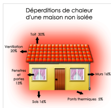
Figure 136 : Schéma des déperditions de chaleur d'un habitat
