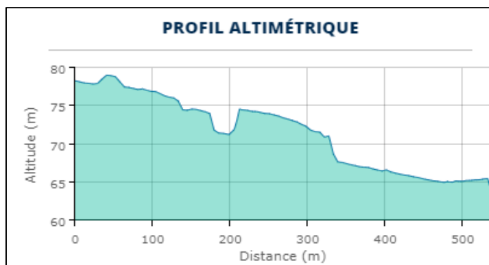
Figure 111 : Profil altimétrique de l'axe de ruissellement N°2.
